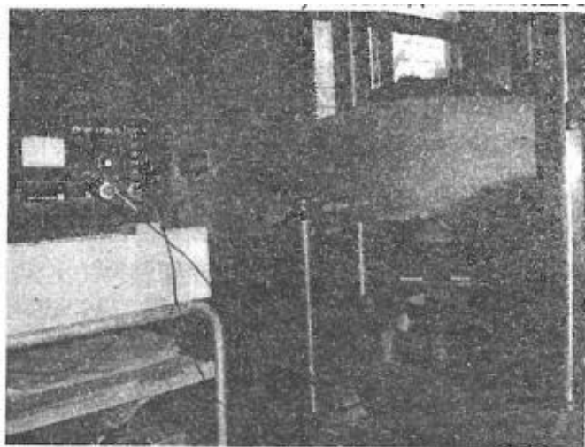
Рис. 1. Нагружение (на прессе ЦДМ-100) и прозвучивание (УК-10 ПМ) призматического образца
