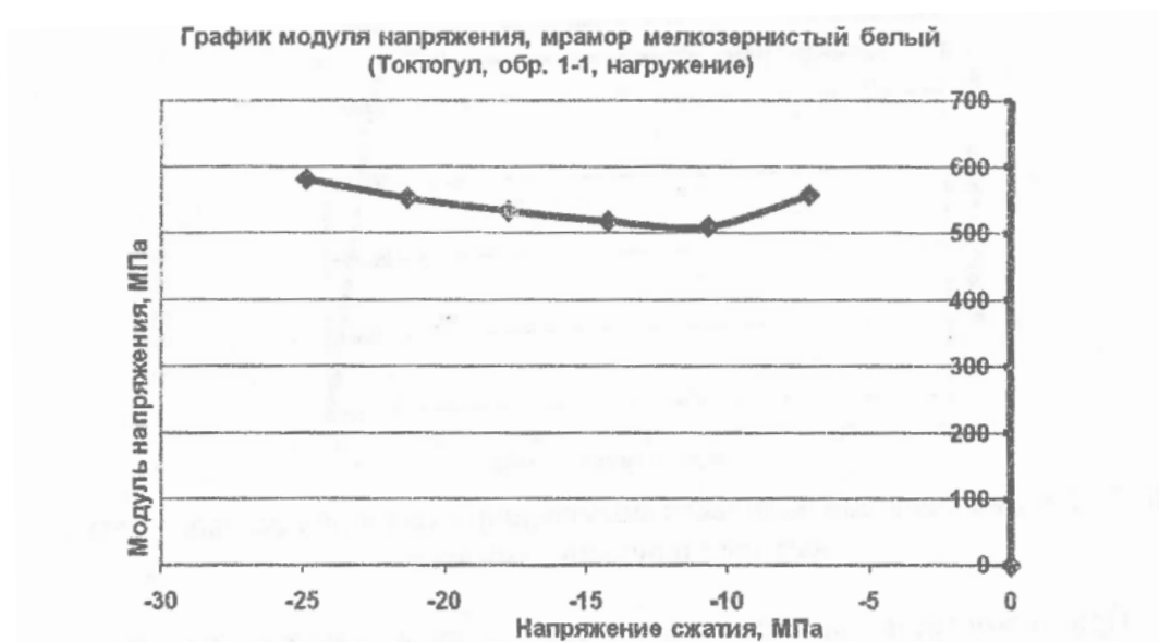
Рис. 11. График значений волнового модуля напряжения при разных уровнях нагрузки одноосного сжатия (мрамор тонкозернистый, Токтогул, образец № 1-1)
